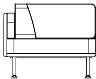
30003 Corner module W 90,0 cm / 35.4" D 90,0 cm / 35.4" H 64,5 cm / 25.4" SH 39,5 cm / 15.6" Net/Gross weight 23,5 kg / 33,1 kg Volume 0,61 m 3 Unit 1 pc
